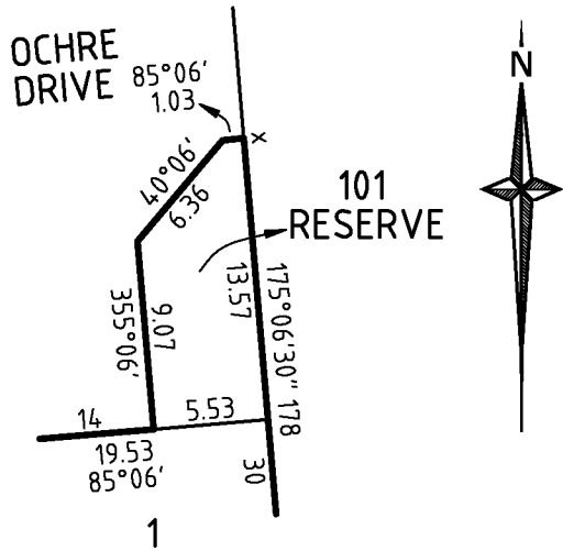
ENLARGEMENT E1
