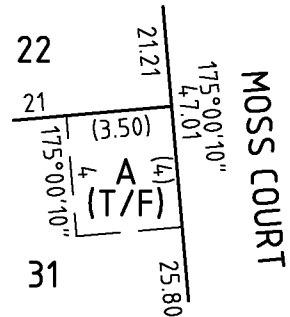
ENLARGEMENT E2
