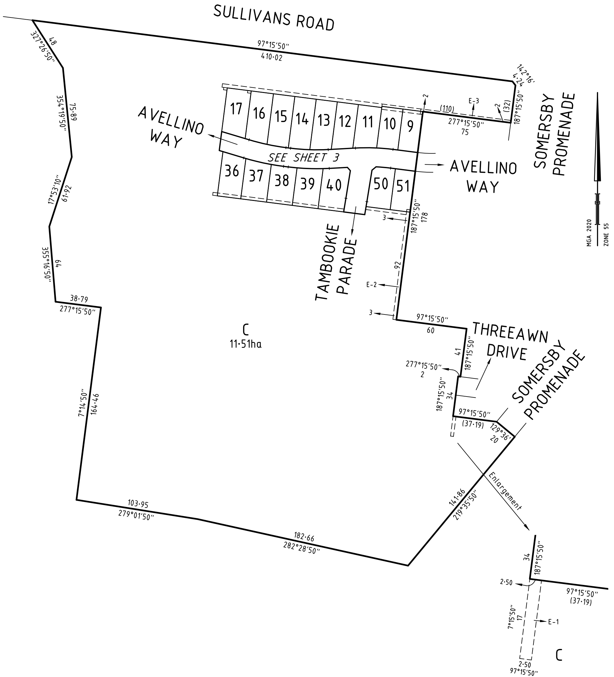
ENLARGEMENT SCALE 1:500
